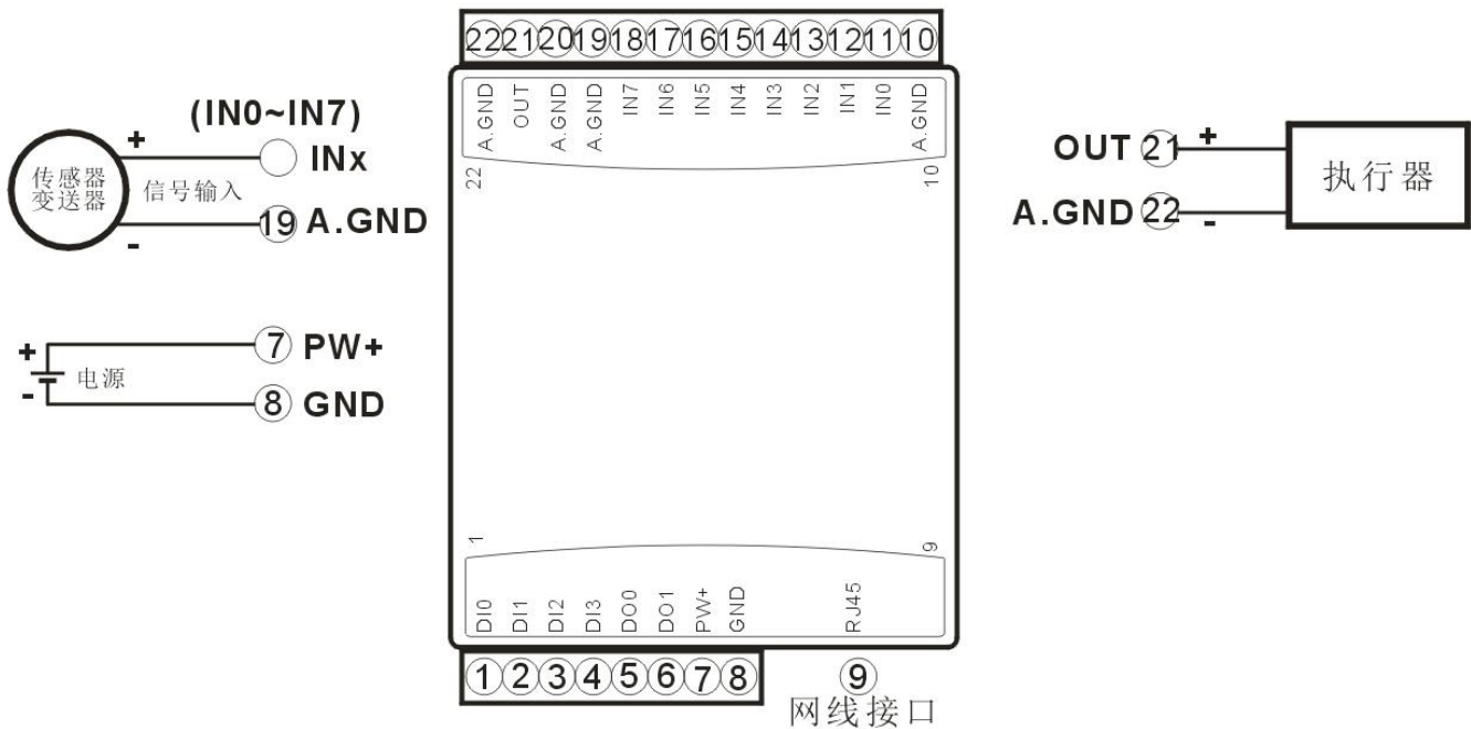
图 5 SAR80 模块接线图
