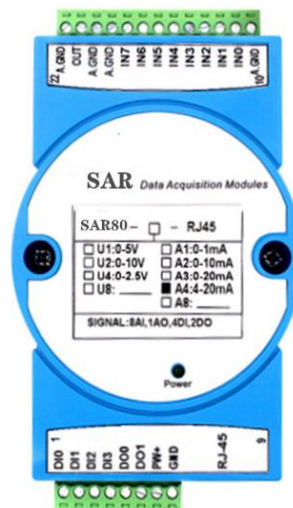
SAR80外观图
