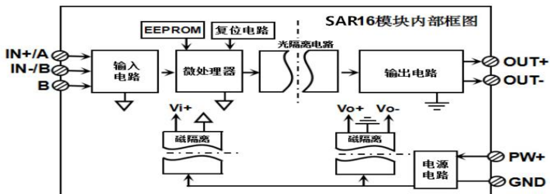
图 2 产品原理框图
